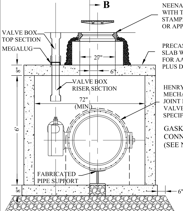
SECTION A-A
